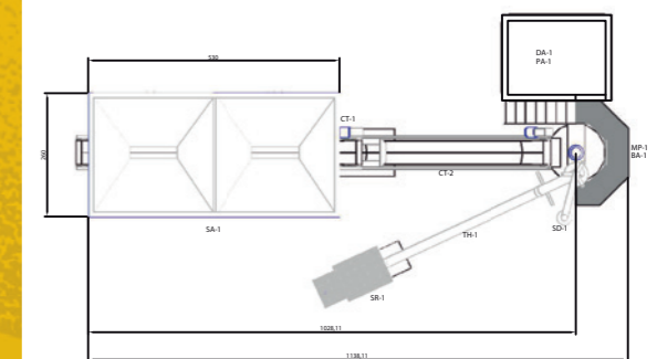
Planta Baixa
